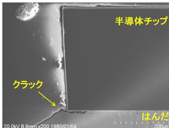
熱ストレスによる故障の事例 半導体チップ接合部のはんだクラック
