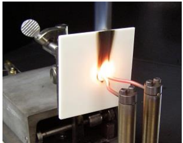
グローワイヤー試験
