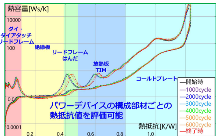
過渡熱抵抗測定機(T3Ster)による熱抵抗測定結果の例
