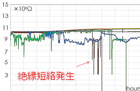
絶縁抵抗値プロフィール
