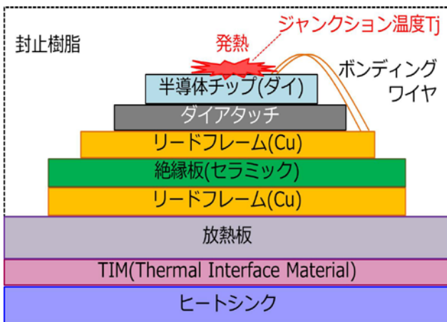
パワーデバイスの構造模式図
